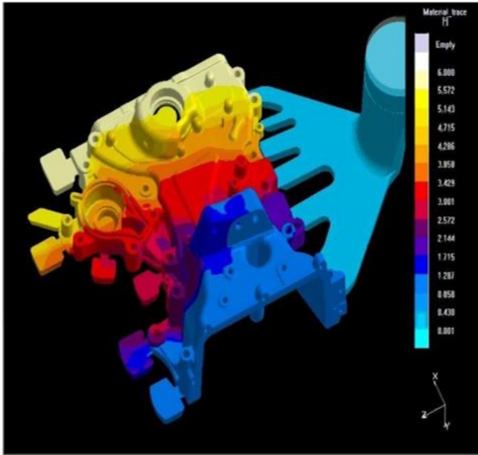
模流分析 Mold flow Simulating
