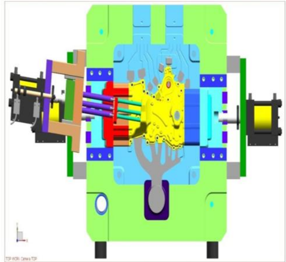
模具方案 Mold Design
